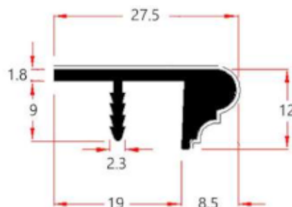
LP 1219 T
