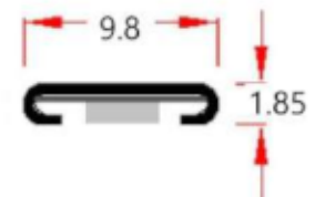
ABS CLIPO 24138
