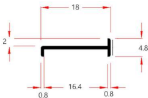
PCA 5164 PL
