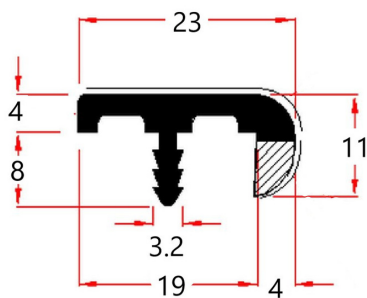
PRONEZ 1119 T BICOL
